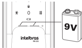
Bateria 9V
